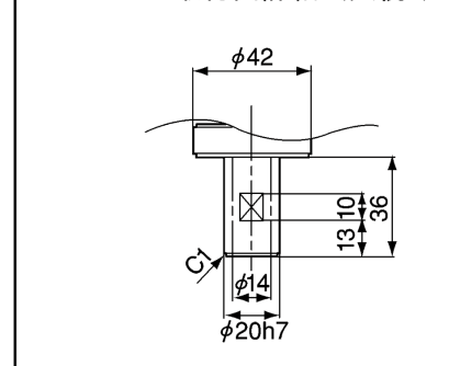
ツール取付面詳細 (矢視D)
