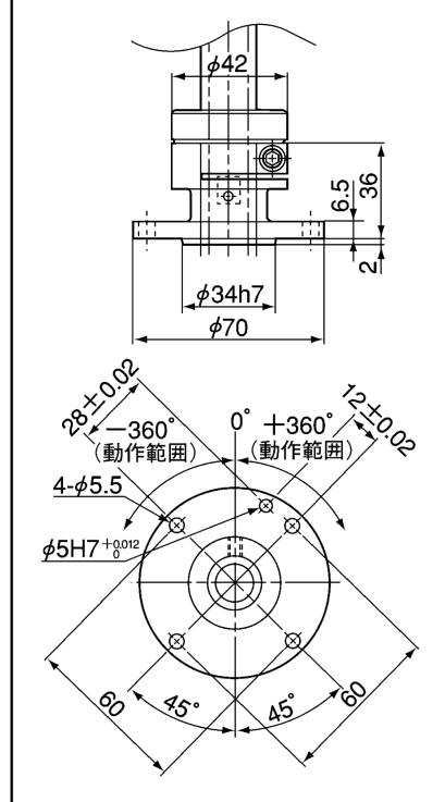
フランジ (オプション) 取付図
