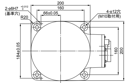
ベース取付面 (上面より)
