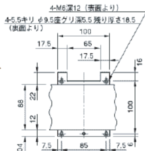
Ⓐ 矢視
